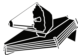
JWST
