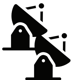
ALMA
