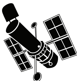
HST
