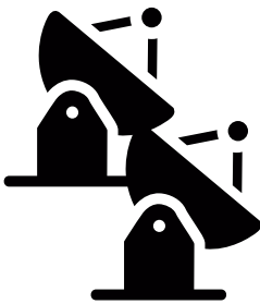
ALMA
