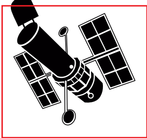
HST
