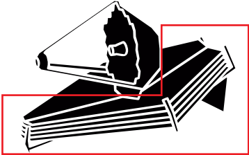
JWST
