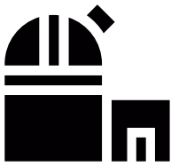
DESI
